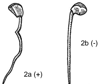
Fig. 2 Cotyledon "knee".
