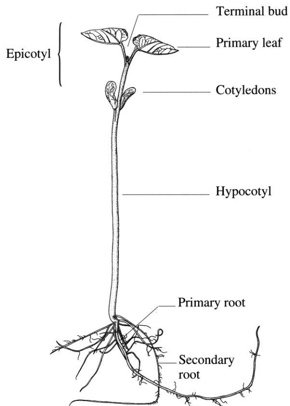
Fig. 1 Bean.
