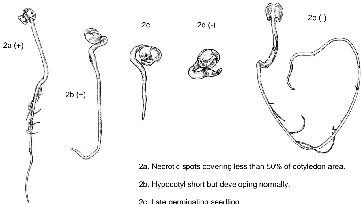
Fig 2. Brassica
