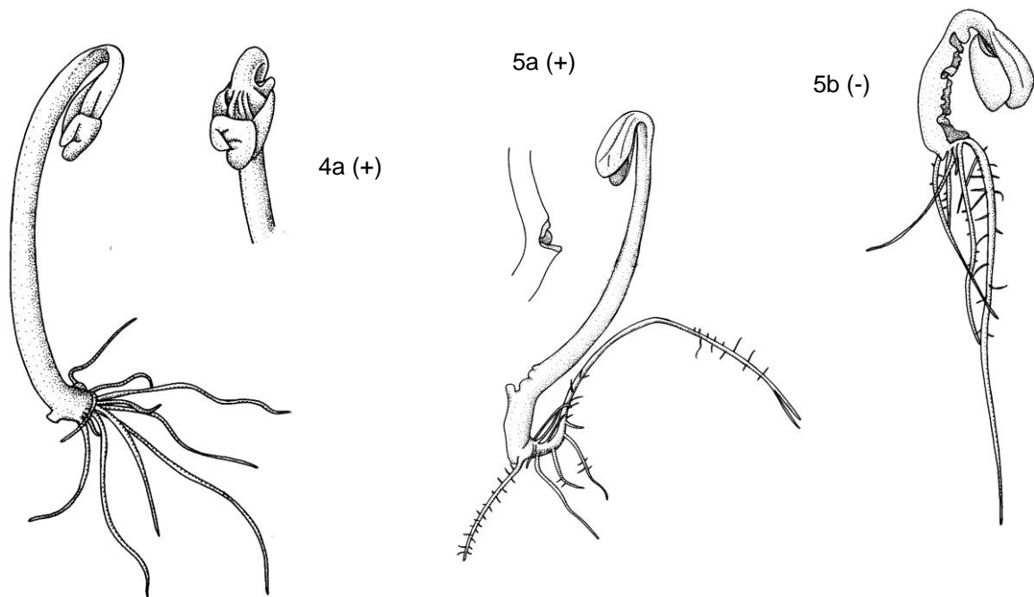
Fig. 5 Hypocotyl lesions.
